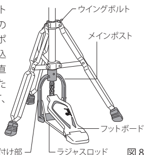
ラジャスロッド取り付け部 ラジャスロッド 図 8
